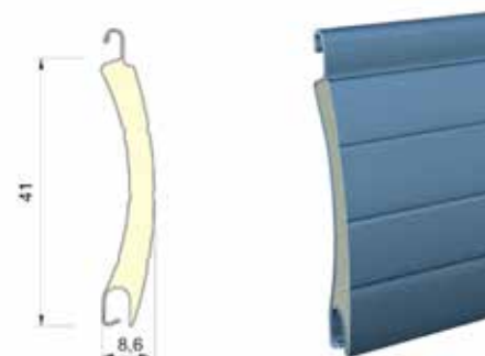
LAMELLE BP41R
